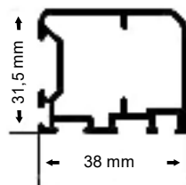
Perfil Hoja Shutter Profile Fiche Profil Blattprofil
